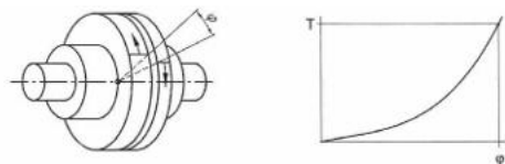
Banda de resorte de torsión y ángulo de torsión
